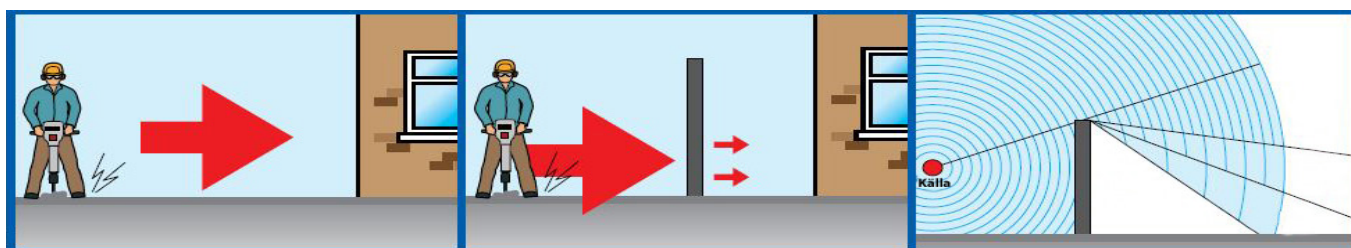
Spridning av ljudvågor från källa, med diffraktion & spridning av ljudvågor
