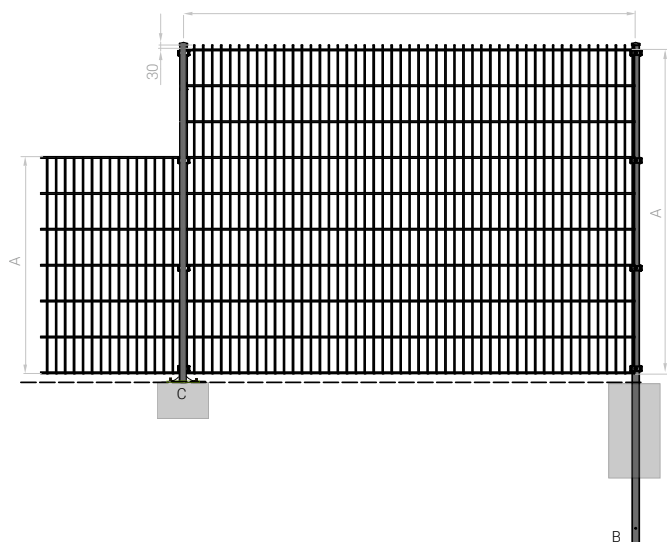
Vertikalt vänd panel
